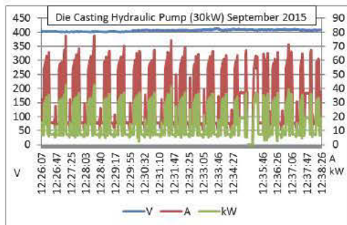
Inverter : 32Hz
