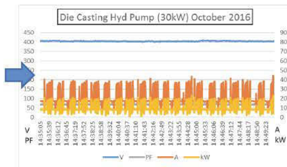
Inverter : 28Hz
